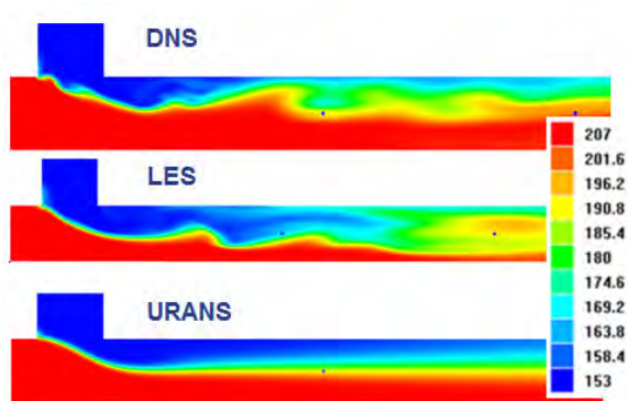
Рис. 13. Мгновенное распределение температуры в плоскости симметрии тройника, полученное в расчетах FV для режима I в различных подходах (цветная версия рисунка доступна в электронной версии на сайте журнала)
