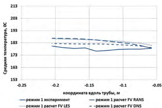
Рис. 11. Средняя температура натрия в контрольных точках T1–T10 на поверхности тройника, полученная в расчетах FV для режима 1
