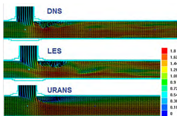
Рис. 14. Мгновенное поле скорости в плоскости симметрии тройника, полученное в расчетах FV для режима I в различных подходах (цветная версия рисунка доступна в электронной версии на сайте журнала)
