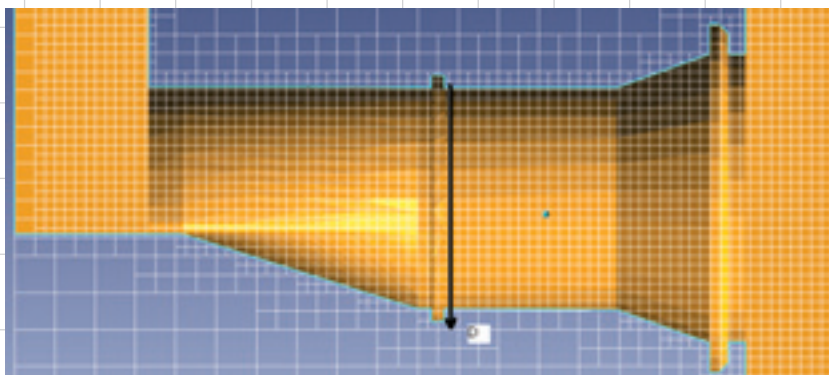
Рис. 3. Расчетная сетка
