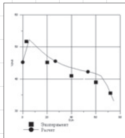
Рис. 8. Эпюра скоростей в сечении 6 (вертикальное)
