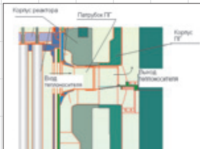
Рис. 1. Конструктивная схема входного участка ПГ
